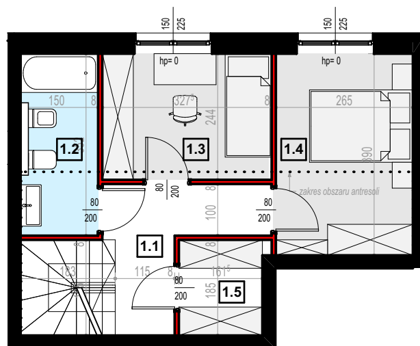
rzut piętra
