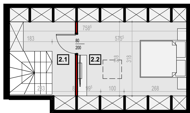
rzut antresoli
