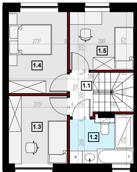
rzut piętra
