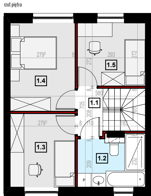
rzut piętra
