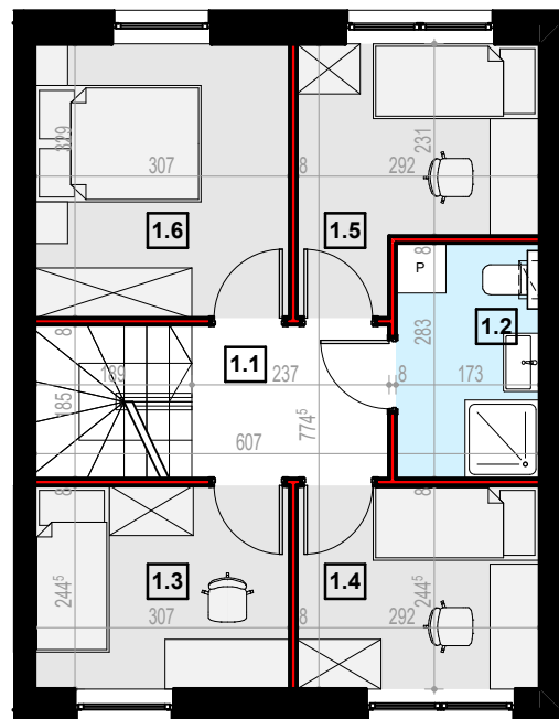
rzut piętra
