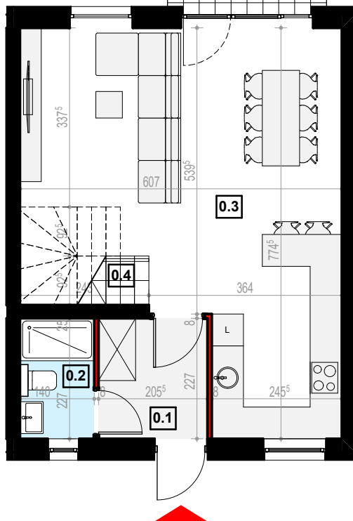
rzut parteru
