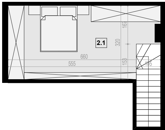
rzut antresoli
